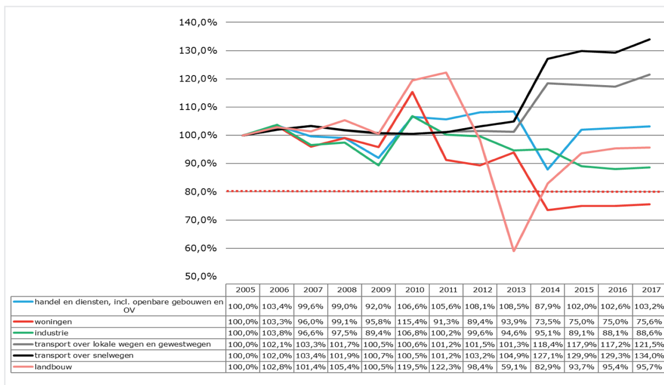
Figuur 12.2.2: Evolutes CO 2 -uitstoot per sector (tCO 2 %), 2005-2017
