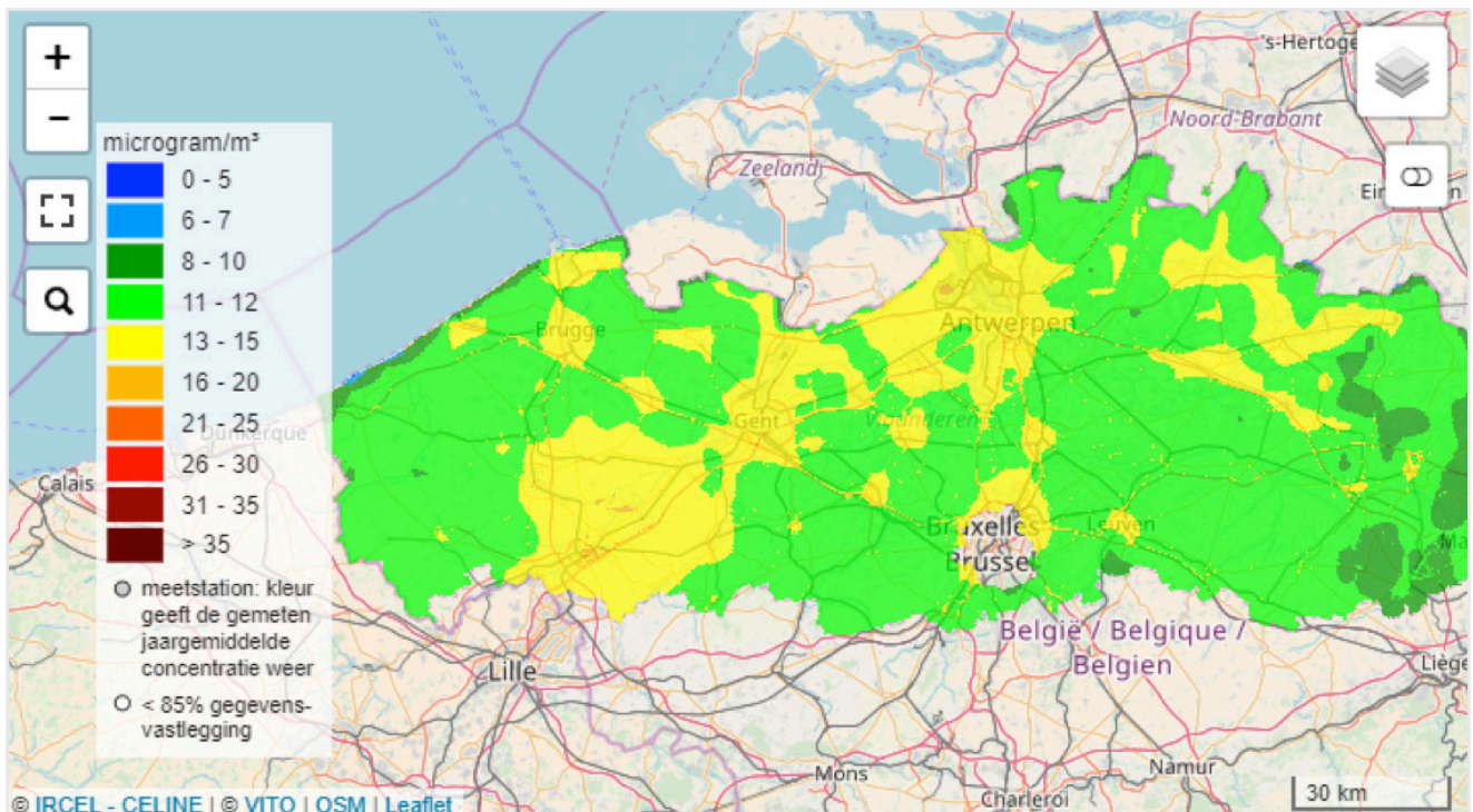
Kaart 7.1.1.1: Fijn stof PM 2,5 interpolatie in Vlaams Gewest, 2016.
